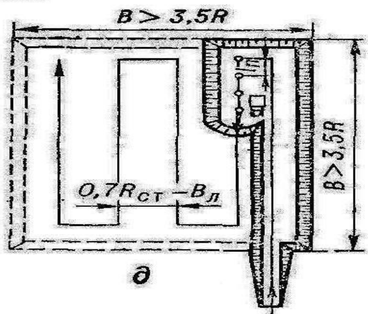
Рисунок 12. Разработка грунта экскаватором прямая лопата
