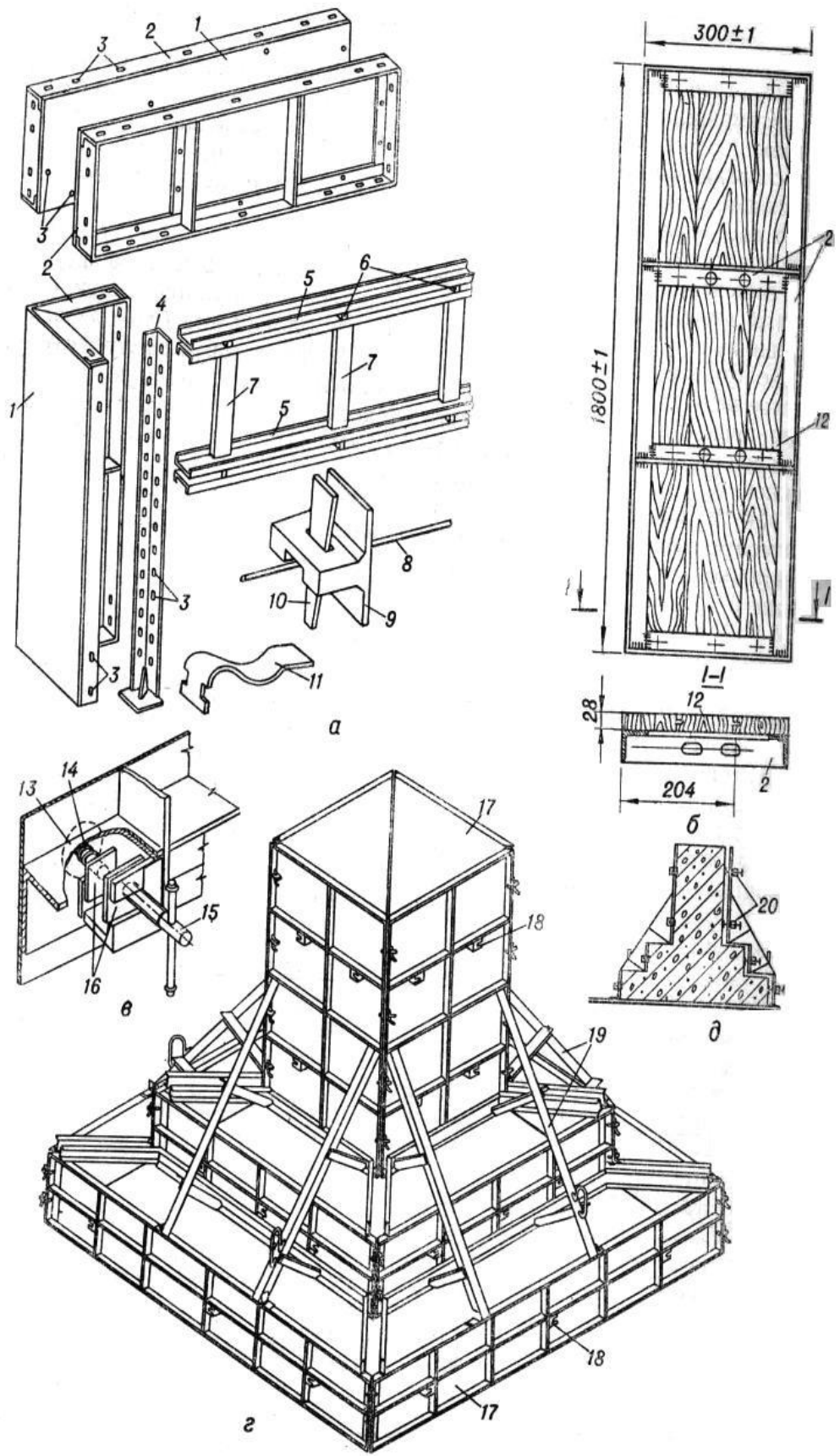
Рисунок 16. Опалубка типа “Монолит” и блок-форма
